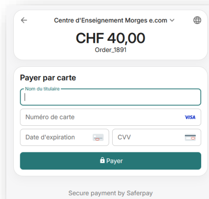
Exemple VISA
