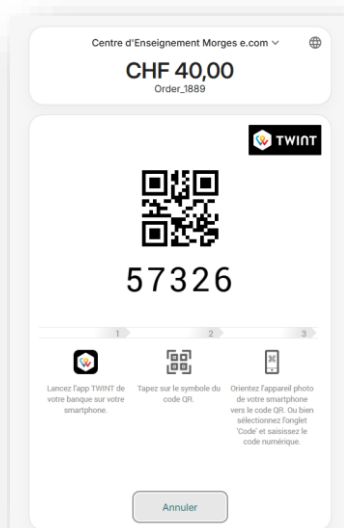
Exemple TWINT
